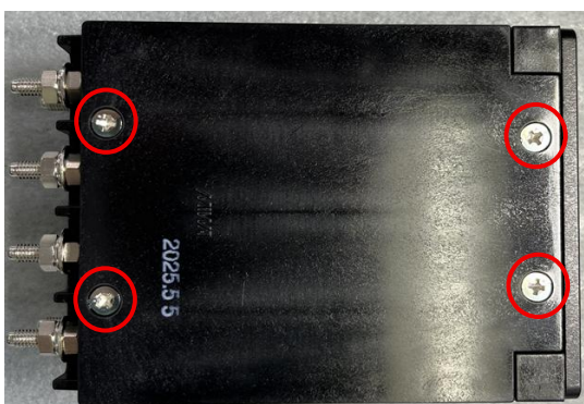
テストターミナル上面、底面の皿ネジ
